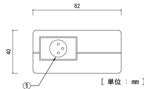
側面図 3
