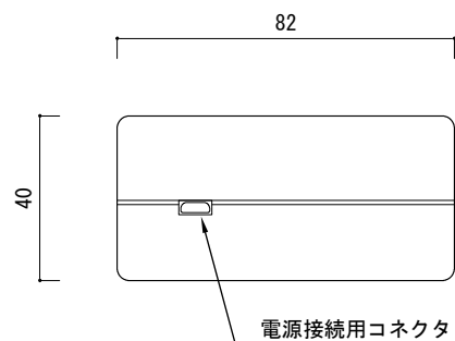
側面図 1
