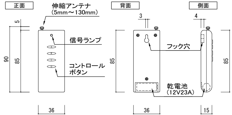
付属リモコン (非防水)
