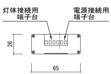
側面図 3
