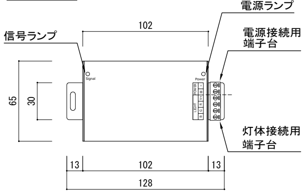
上面図
