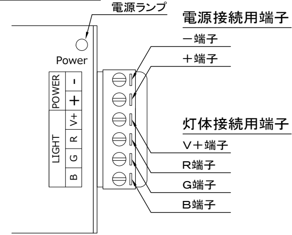
端子台 拡大図
