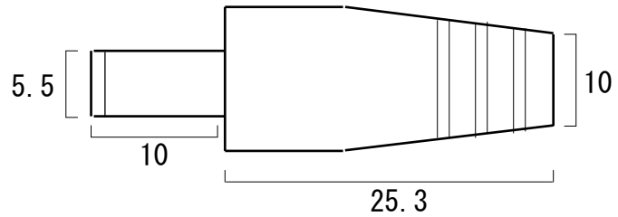
コネクタ拡大図
