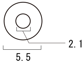
プラグ先端拡大図
