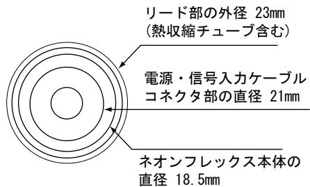
リード部断面拡大図
