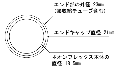
エンド部断面拡大図
