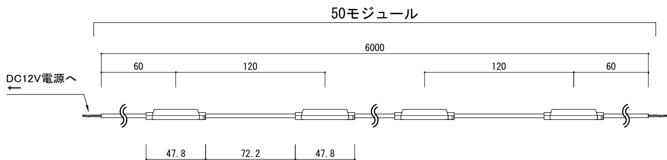
側面図
