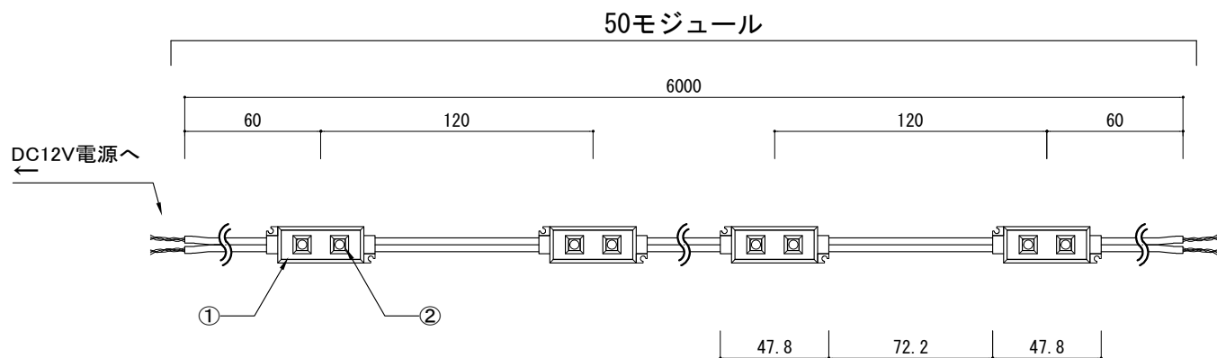
上面図
