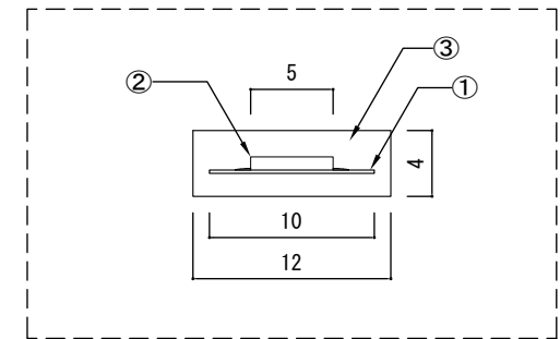
断面拡大図
