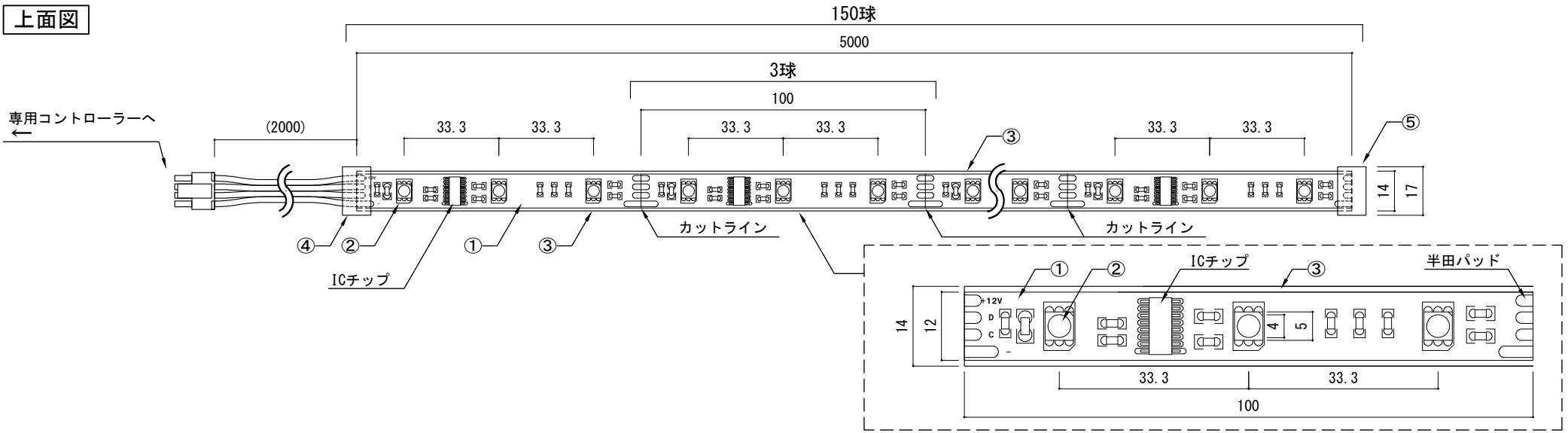
拡大図
