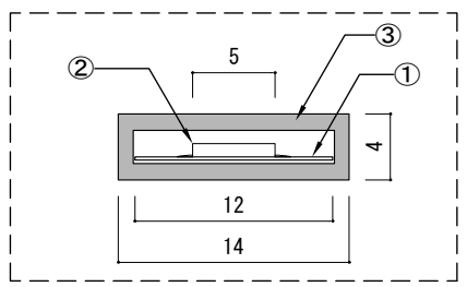
断面拡大図
