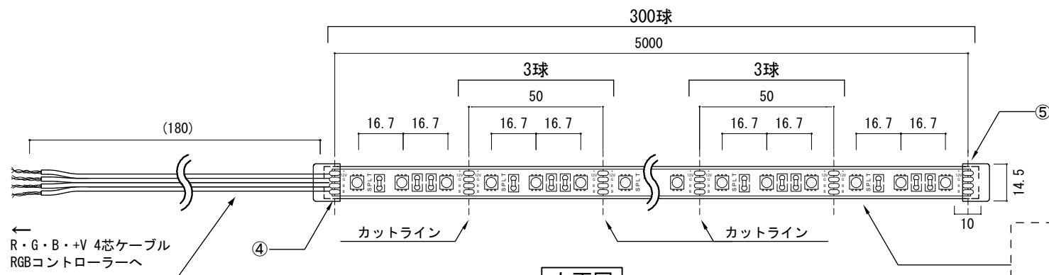
上面図
