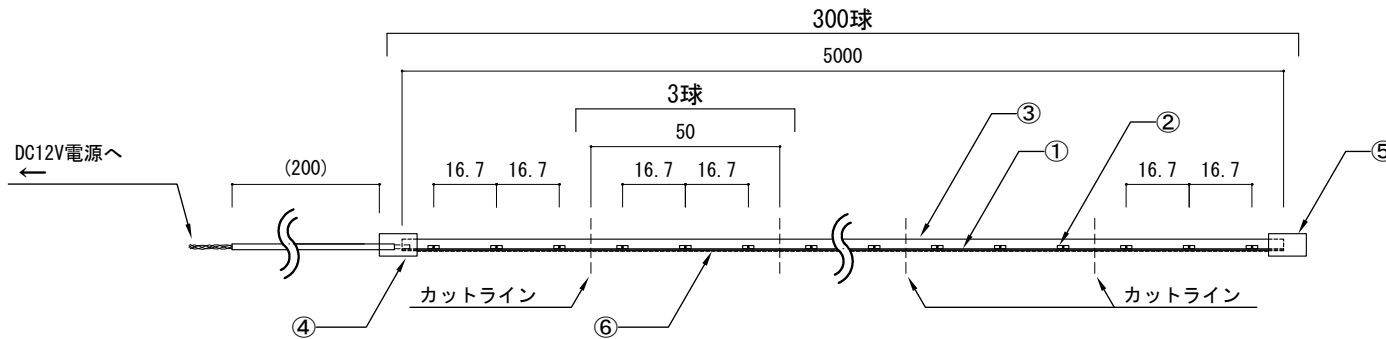
側面図
