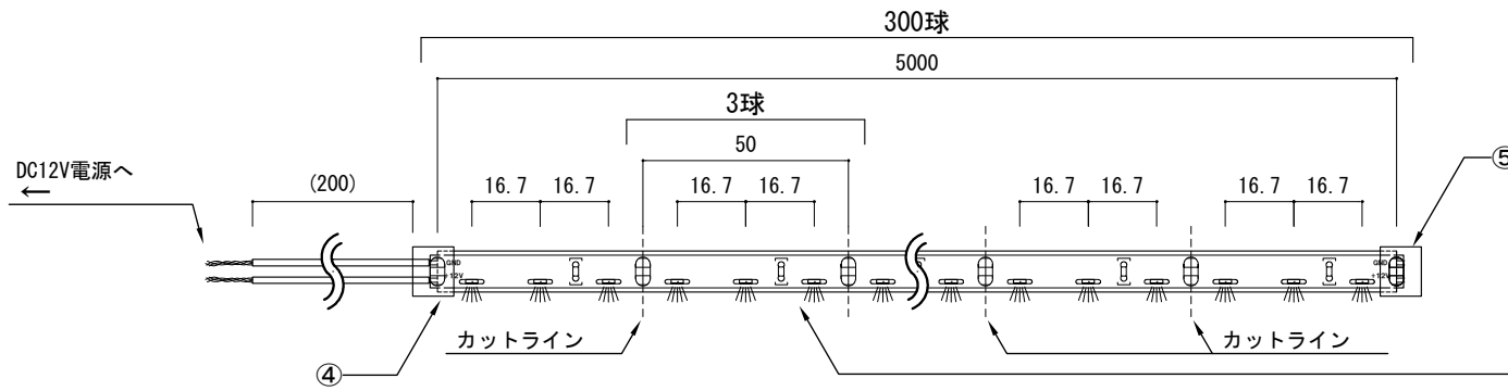
上面図
