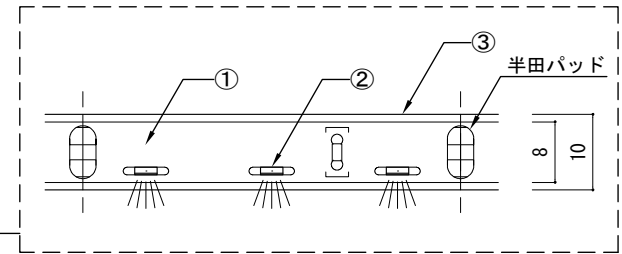
拡大図
