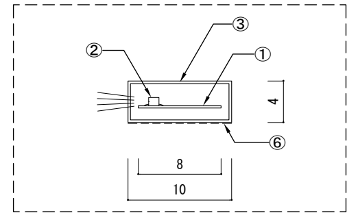
断面拡大図
