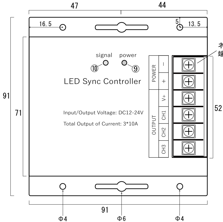
本体 上面図
