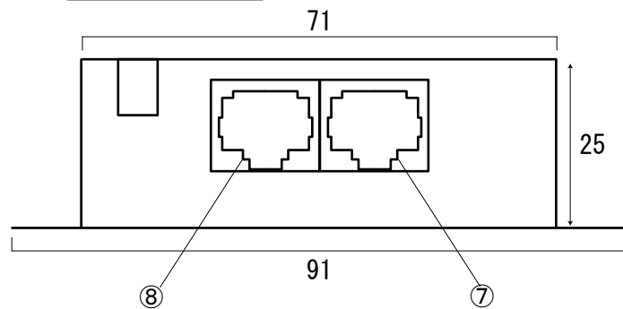
本体 側面図2
