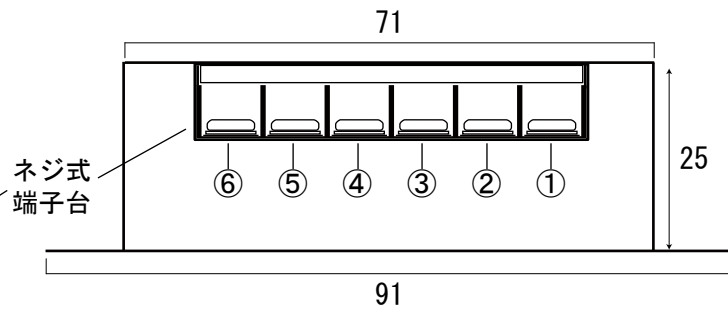
本体 側面図1
