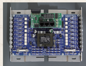
ショータイムコントローラ (基板+ヒートシンク)、液晶付、40A AC16ch 青基板
