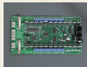
DC コントローラ (基板)、24ch、RGB 用
