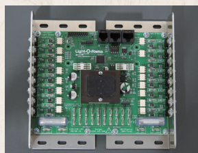
ショータイムコントローラ (基板+ヒートシンク) AC16ch
