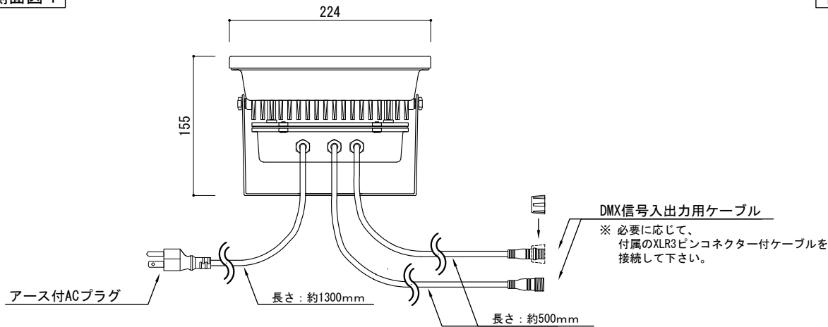
側面図 1
