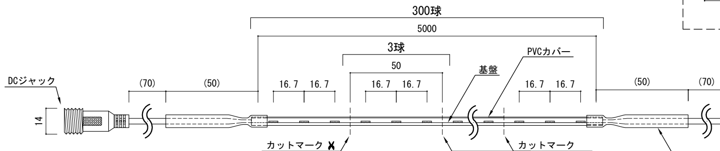
側面図
