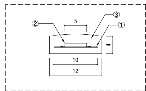
断面拡大図
