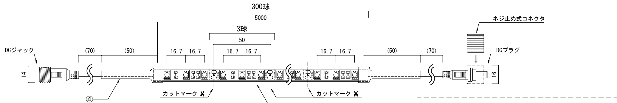
上面図
