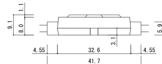
側面拡大図
