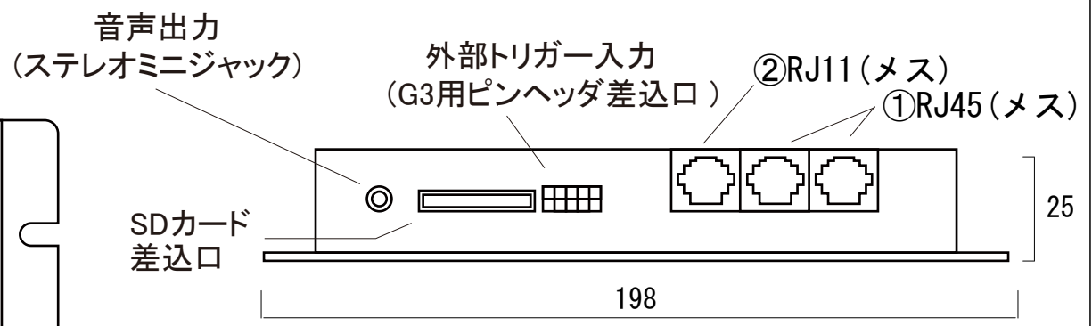
側面図1
