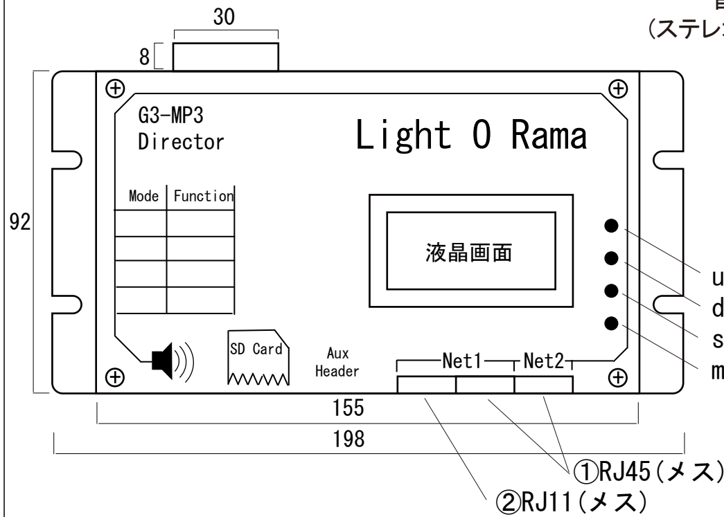
上面図
