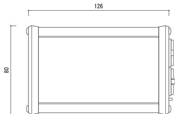
上面図
