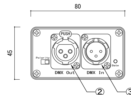
側面図 3
