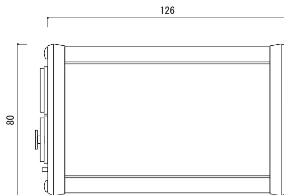
底面図
