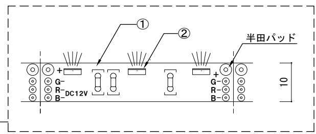
拡大図
