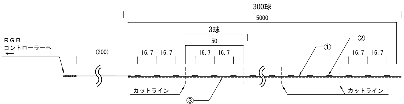
側面図
