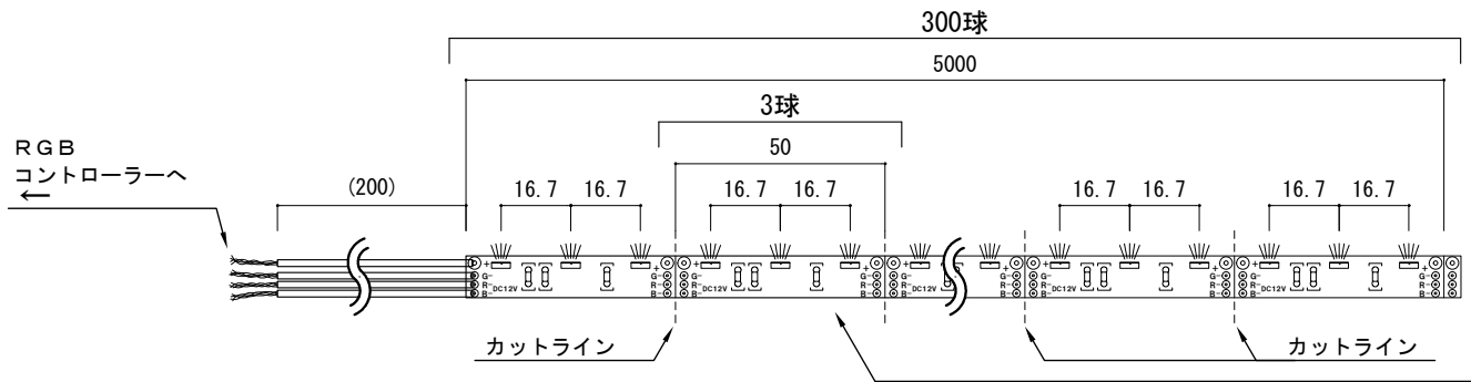
上面図
