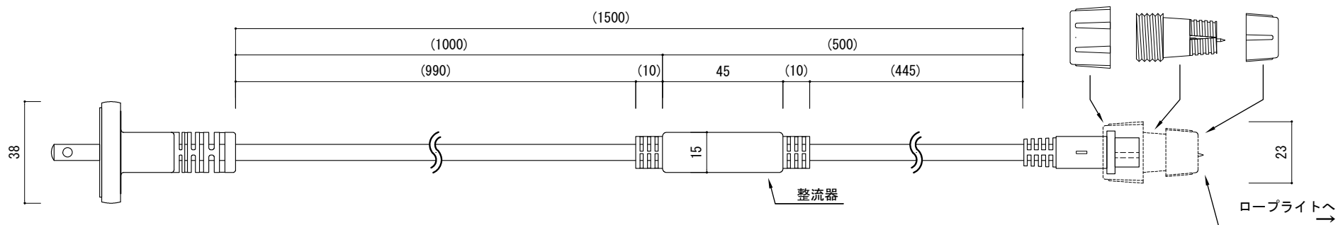
側面図
